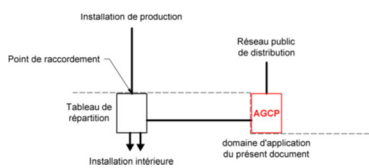
Figure 1 - Limite de l'installation intérieure en cas d'injection du surplus de production sur le réseau public de distribution
